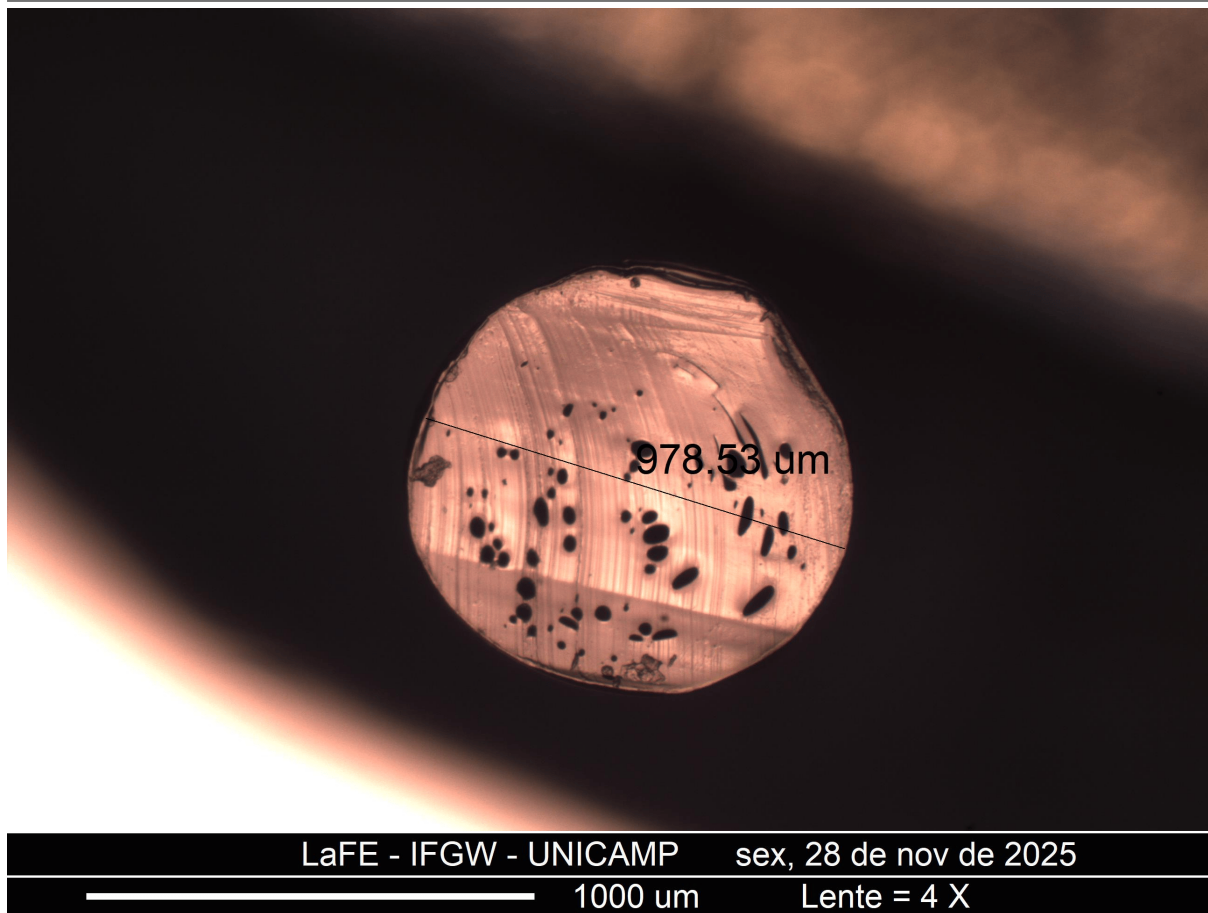
Figura 3: Micrografia da fibra produzida.
